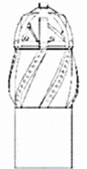
FIG. 7.3 * Nasos-kompresor borularn üçün başmaq * sənaye nümunesinin sol tərəfdən görünüşü
